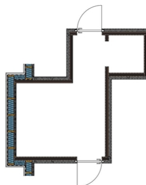
Gekapseltes Treppenhaus
