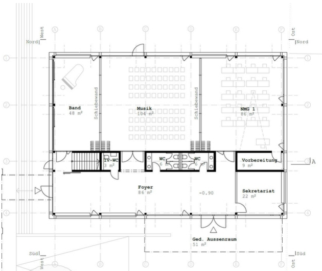
Grundriss Mehrzweckraum
